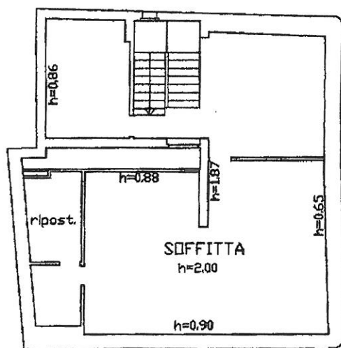
PIANO SECONDO
